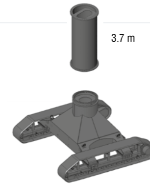
Crawler: XL-undercarriage
